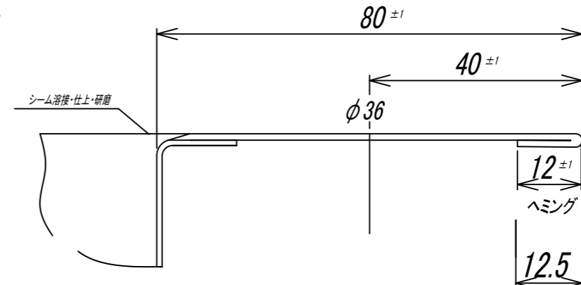
A-A'断面 S=1/1
